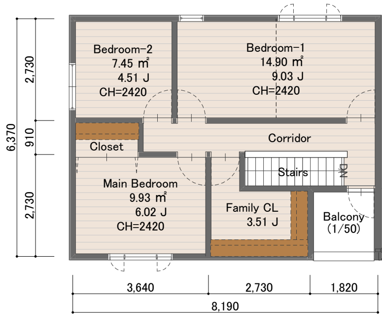
2FL 1:100
