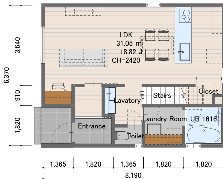
1FL 1:100
