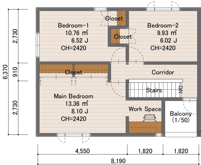
2FL 1:100
