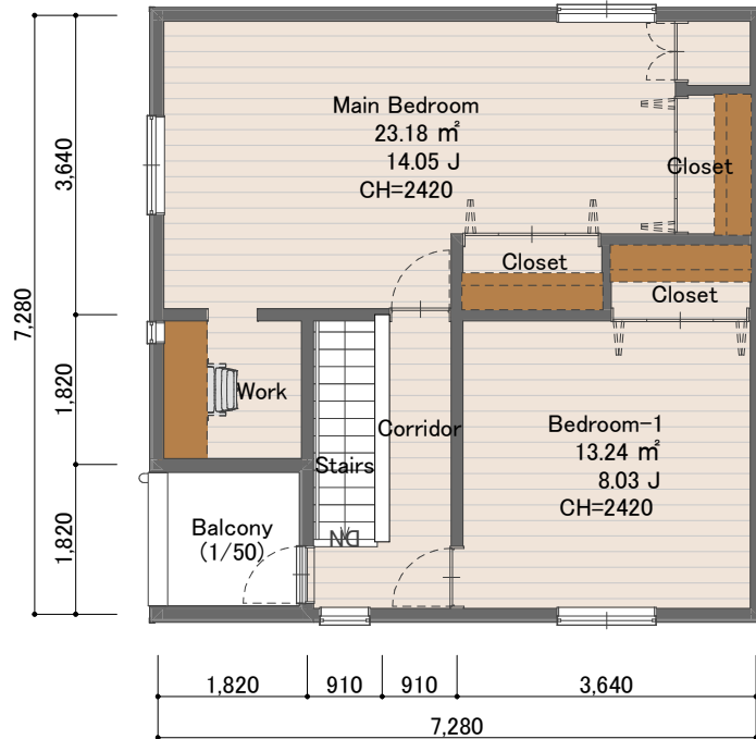
2FL 1:100
