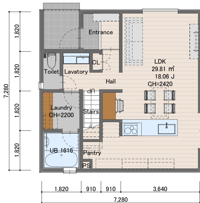
1FL 1:100
