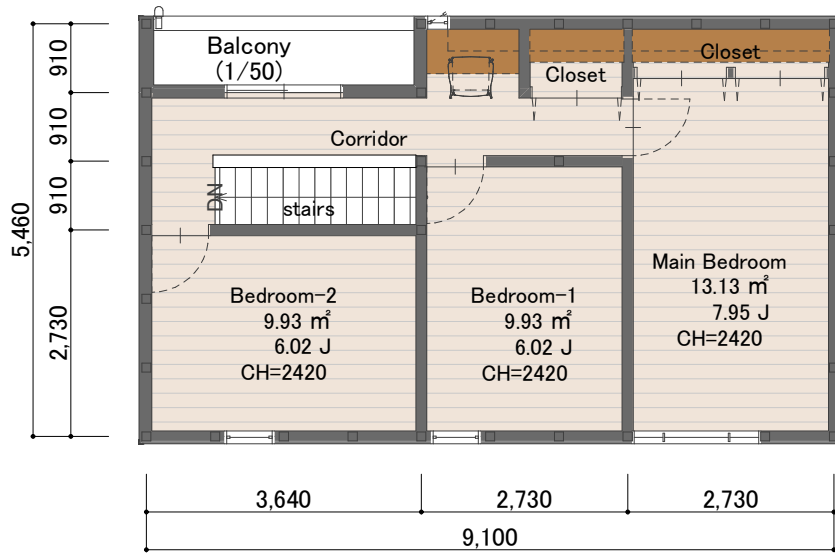
2FL 1:100
