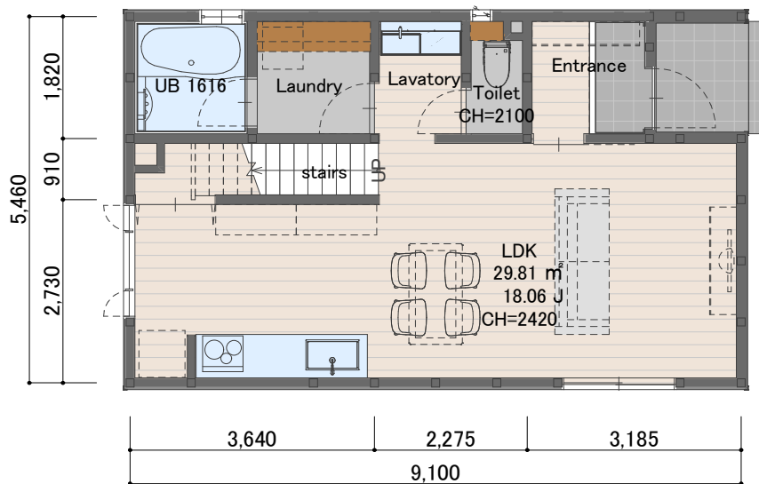
1FL 1:100
